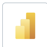
POWER BI
